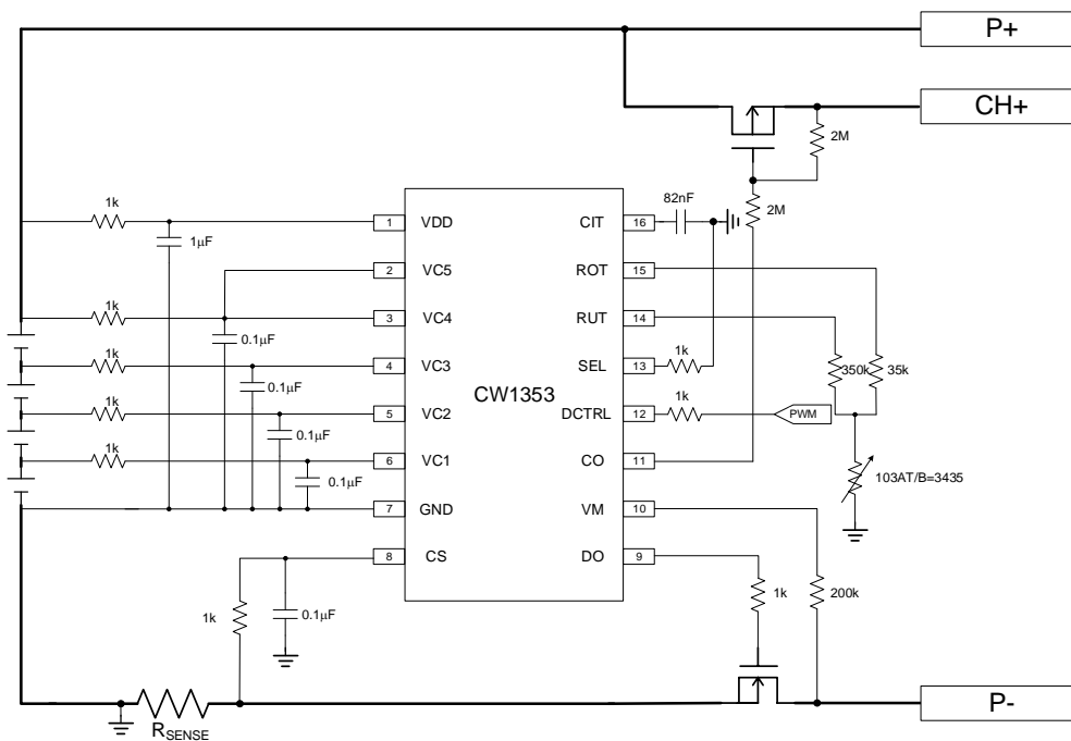
4 串不带均衡功能应用电路
