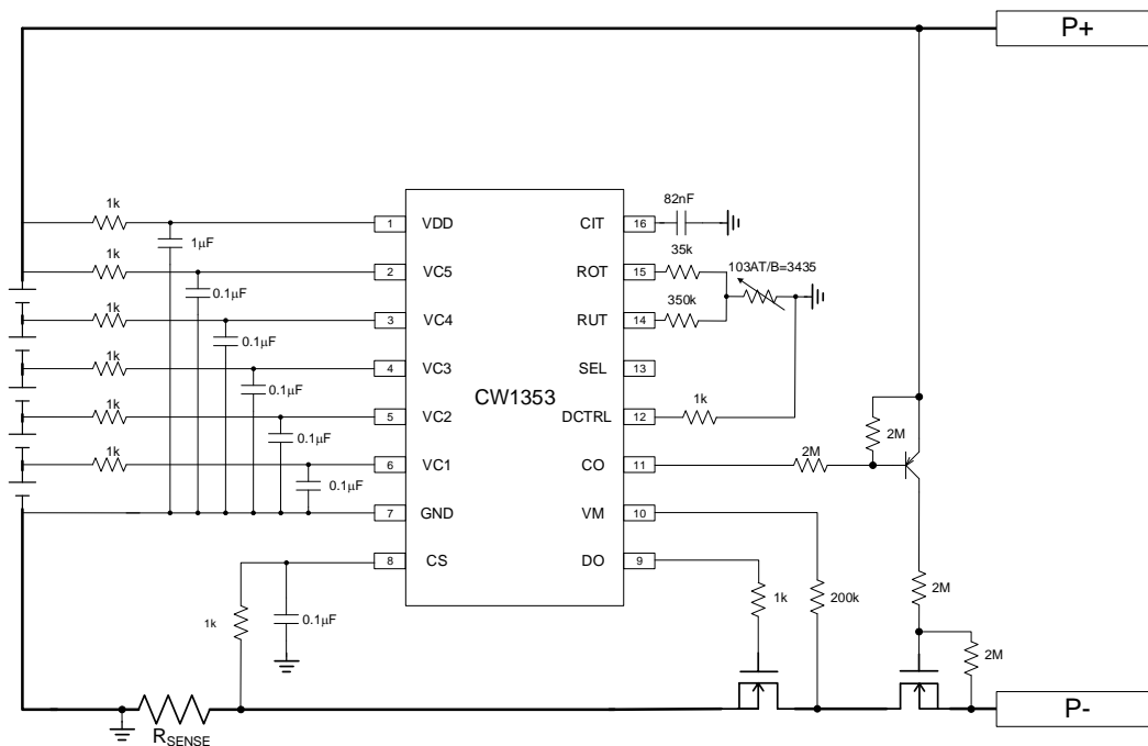
5 串同口应用电路
