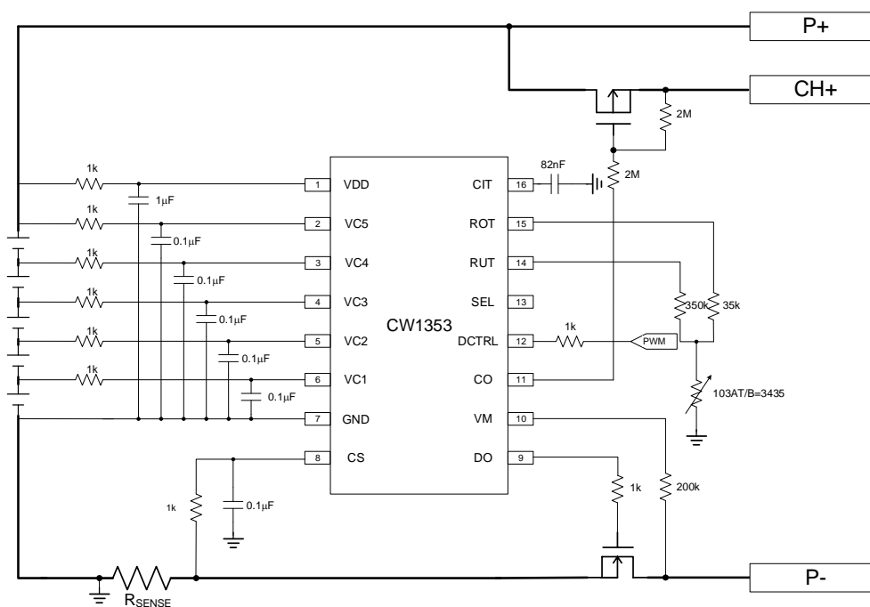
5 串不带均衡功能应用电路
