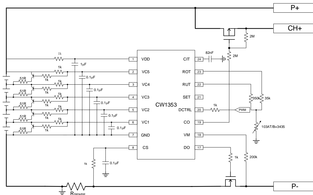
5 串带均衡功能应用电路
