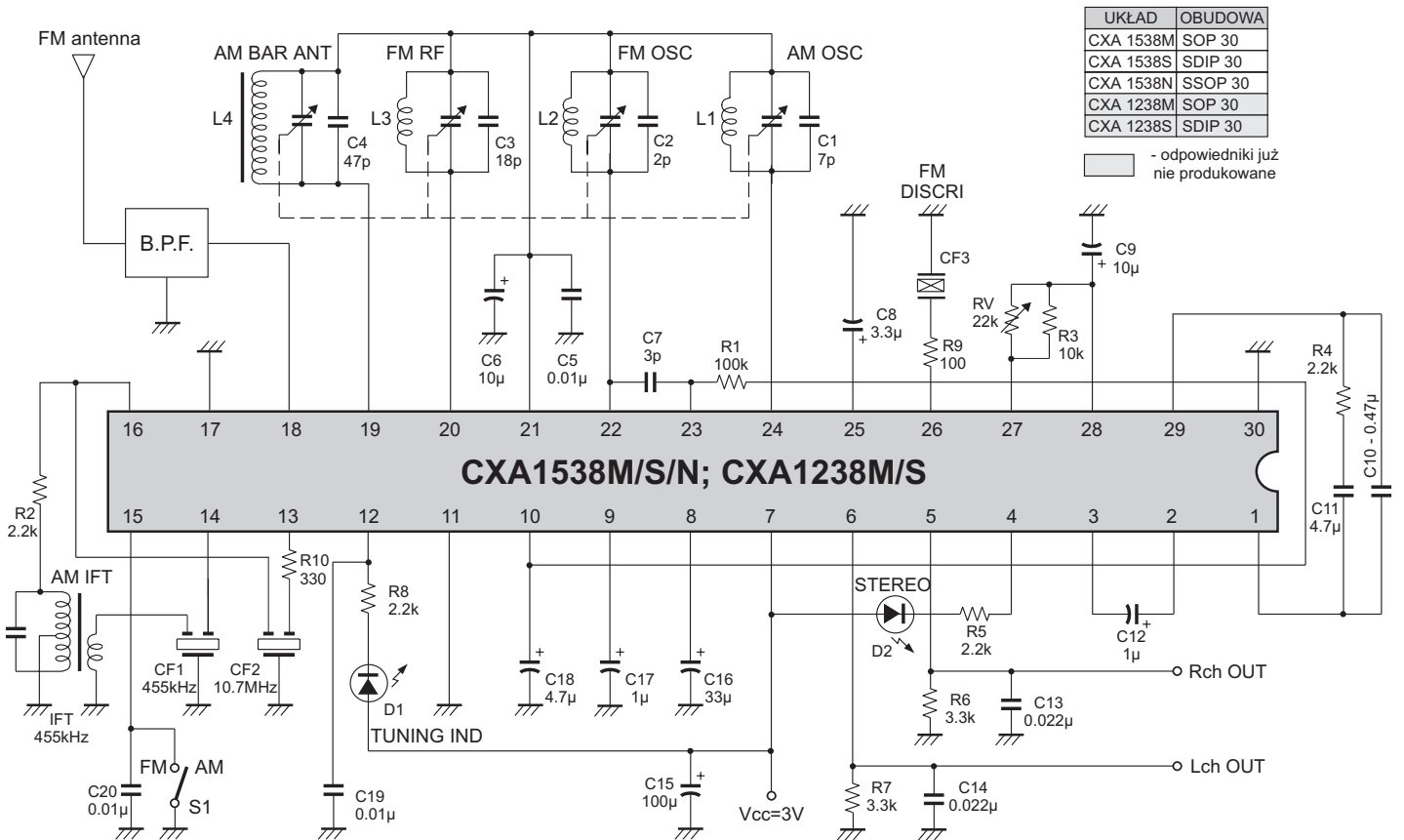
Rys.32. Schemat blokowy i aplikacyjny układu scalonego CXA1538M/N/S.
