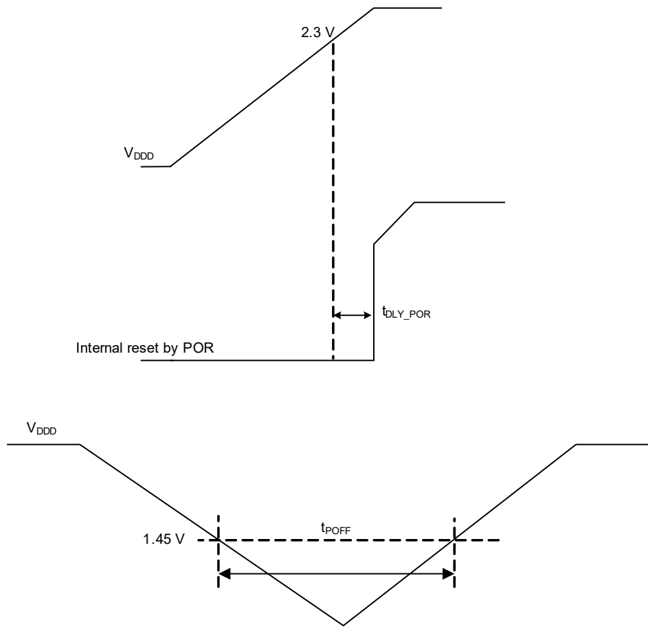
Figure 26-14. POR Specifications
