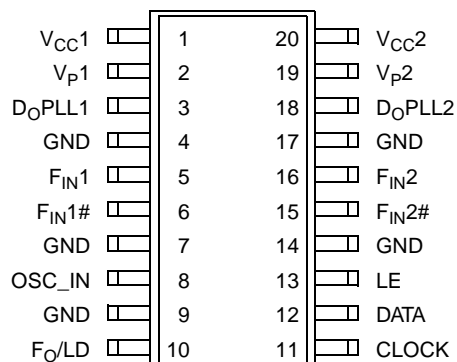
TSSOP
