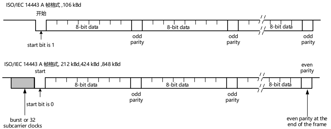
图 7.1 ISO/IEC 14443 A 协议的数据编码和帧格式
