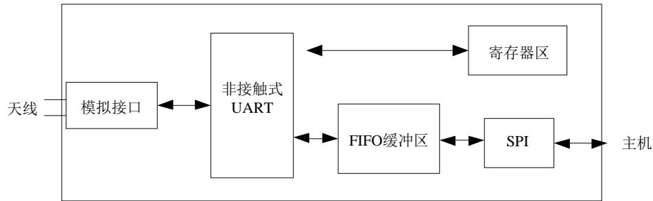
图 5.1 Ci521 简化框图
