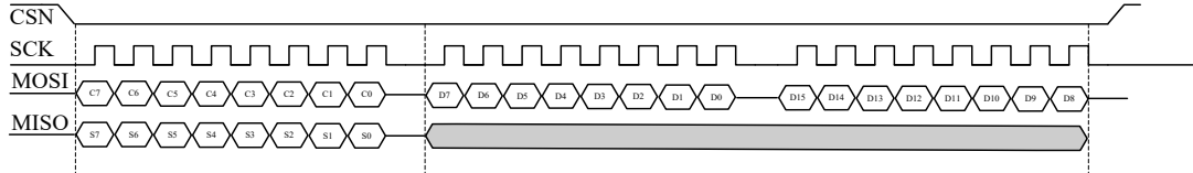
图 7-4 SPI 写操作
