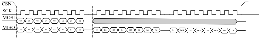
图 7-3 SPI 读操作
