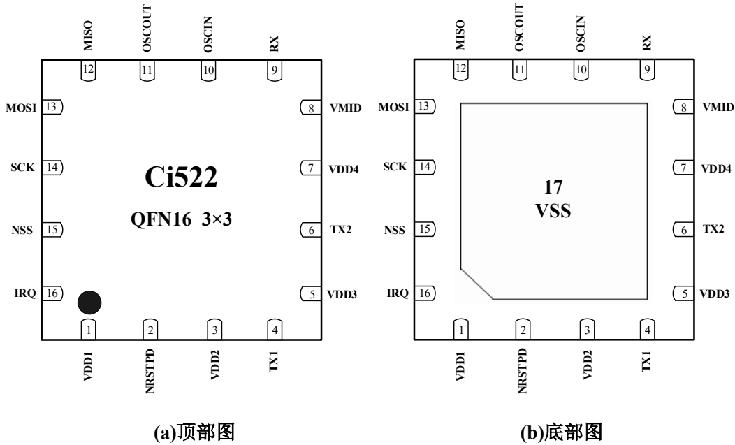
图 6-1 引脚配置图 (QFN16)
