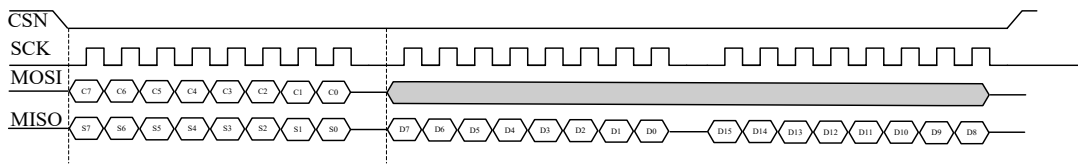
图 7.3 SPI 读
