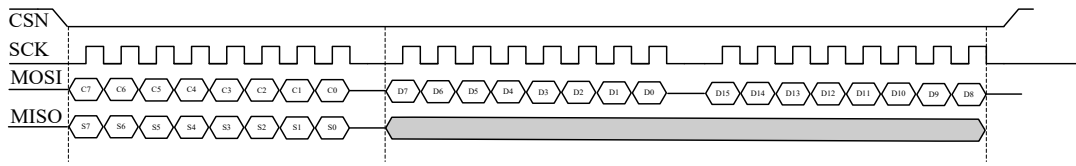
图 7.4 SPI 写
