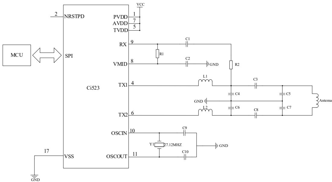
图 10.2 典型应用图-2
