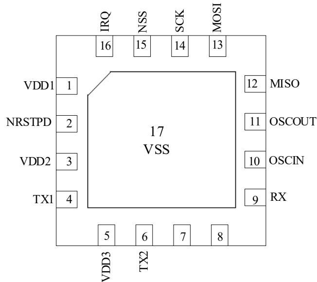
图 6-1 引脚配置图 (QFN16)
