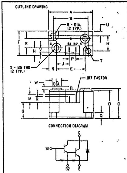
500-600-700 Volt D67DE Outline Drawing
