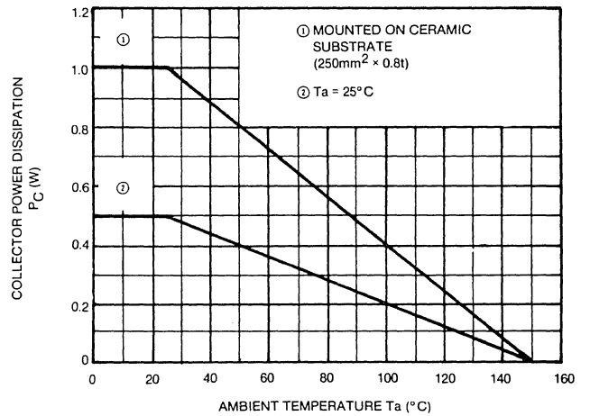
FIG. 6 P_C - T_a
