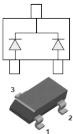
SOT-323
