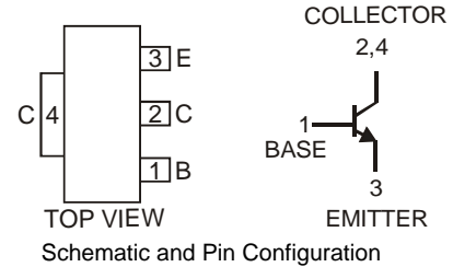
SOT89-3L
