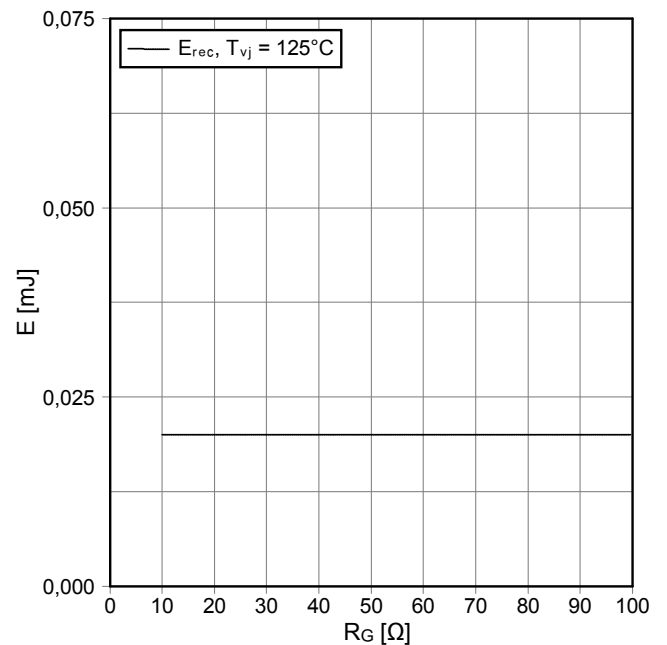
Schaltverluste Diode-Brems-Chopper (typisch) switching losses diode-brake-chopper (typical) E_{rec} = f(R_G) I_F = 24 A, V_{CE} = 300 V
