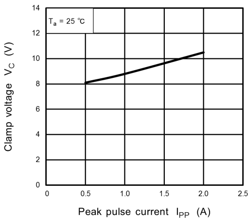
Fig. 5.2.1 V_C - I_{PP}
