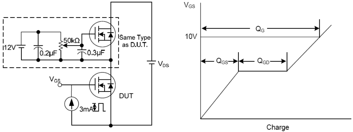
图12. 栅电荷测试
