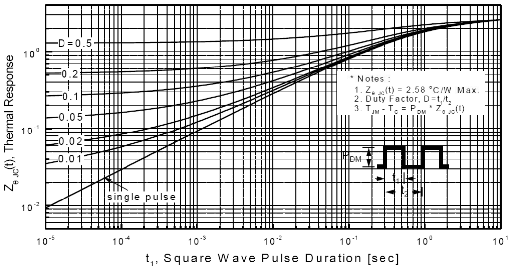
图10. 瞬态热响应曲线(TO-220F)
