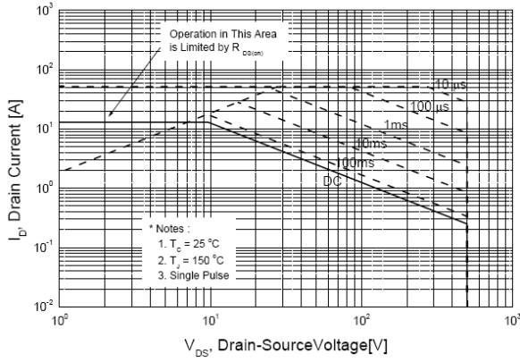
图7. 最大安全工作区
