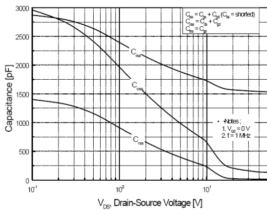
图5. 电容特性曲线 Fig. 5 Capacitance Characteristics
