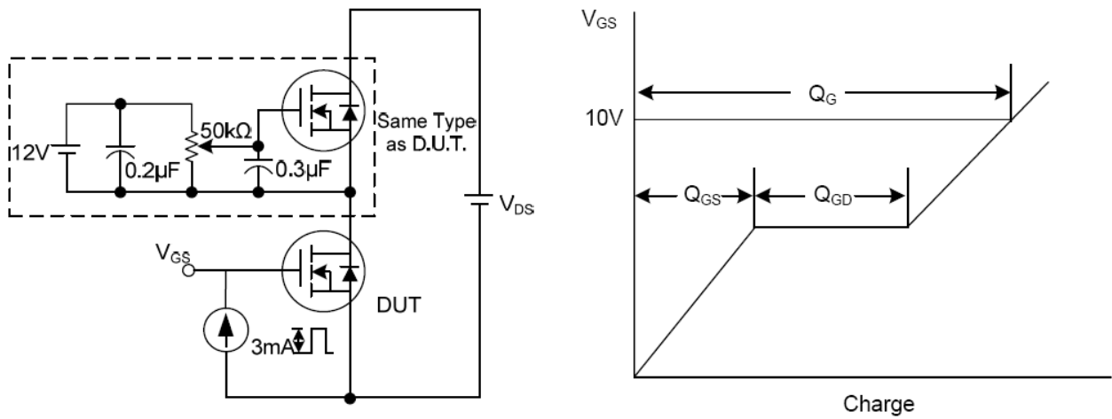
图13. 栅电荷测试
