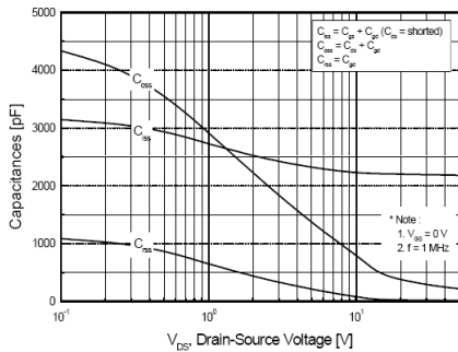
图5. 电容特性曲线 Fig. 5 Capacitance Characteristics
