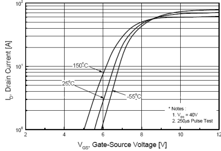
图2. 传输特性曲线 Fig. 2 Transfer Characteristics
