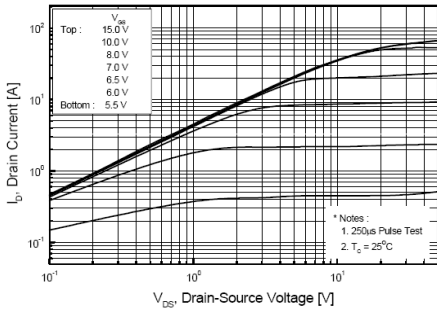
图1. 输出特性曲线 Fig. 1 On-State Characteristics
