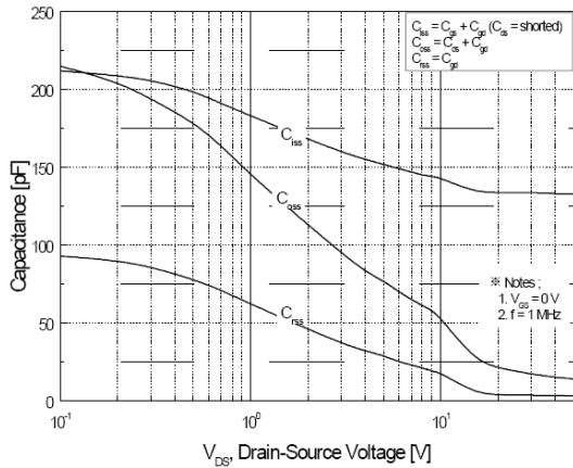
图5. 电容特性曲线
