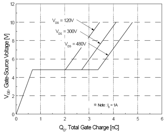
图6. 栅电荷特性曲线
