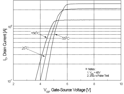
图2. 传输特性曲线
