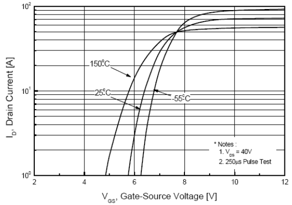
图2. 传输特性曲线 Fig. 2 Transfer Characteristics
