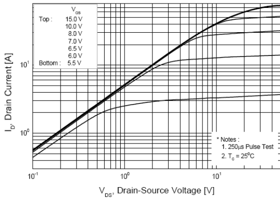
图1. 输出特性曲线 Fig. 1 On-State Characteristics
