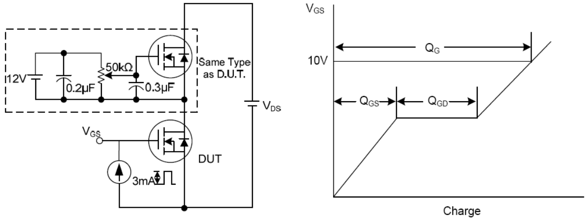
图14. 栅电荷测试
