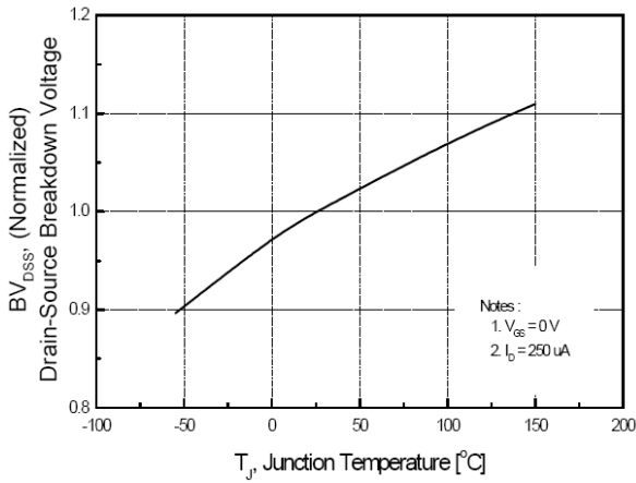
图3. 击穿电压随温度变化曲线
