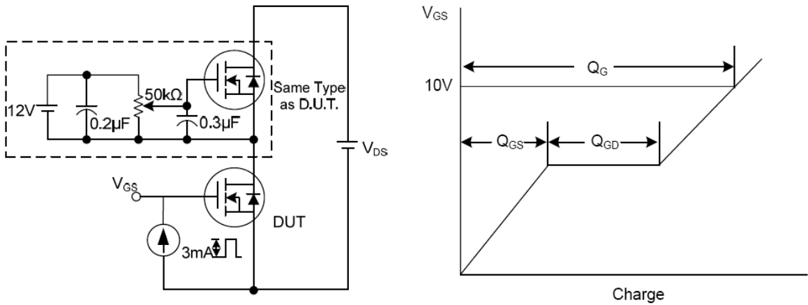
图14. 栅电荷测试
