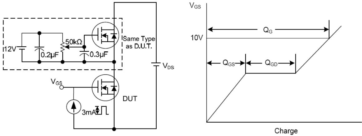
图12. 栅电荷测试
