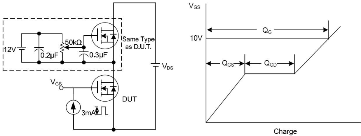
图13. 栅电荷测试
