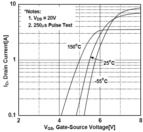
图2. 传输特性曲线
