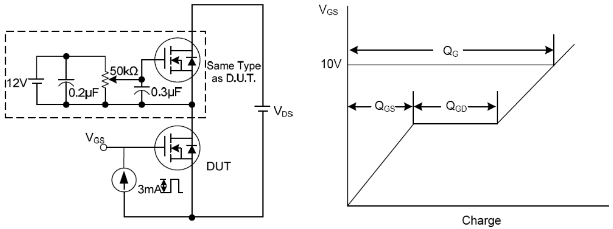
图13. 栅电荷测试
