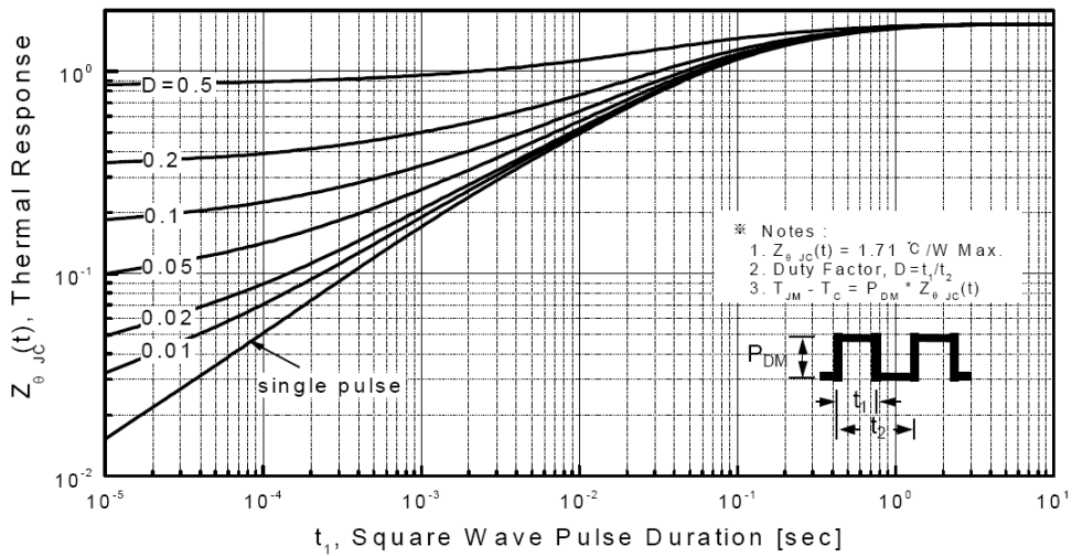
图9. 瞬态热响应曲线(TO-220)
