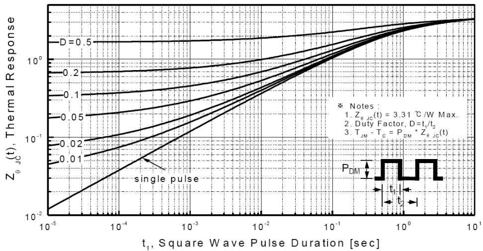
图10. 瞬态热响应曲线(TO-220F)
