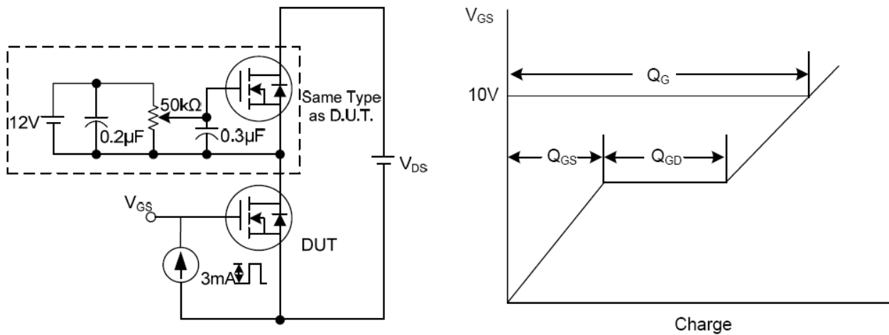
图12. 栅电荷测试
