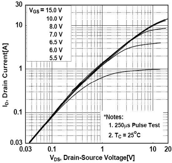
图1. 输出特性曲线
