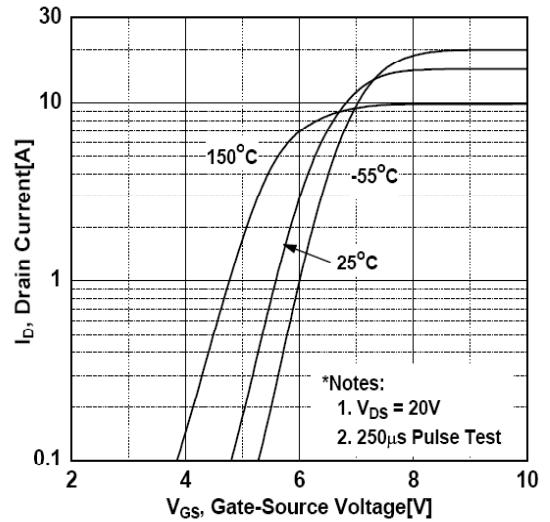
图2. 传输特性曲线
