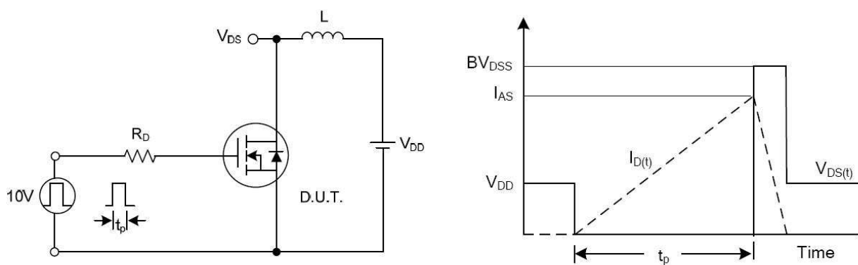
图14. 雪崩能量测试
