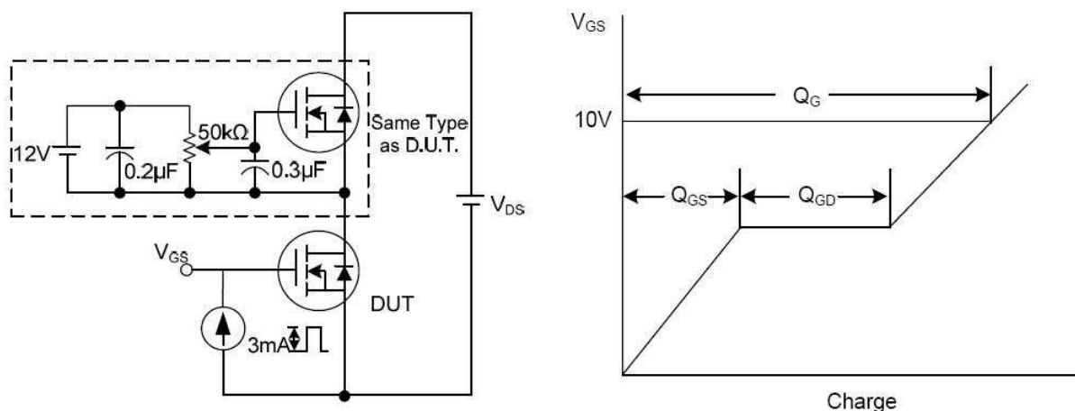
图13. 栅电荷测试
