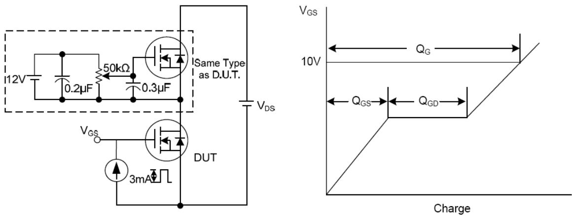
图11. 栅电荷测试
