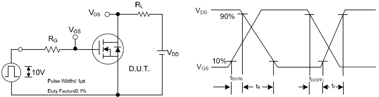
图11. 开关特性测试
