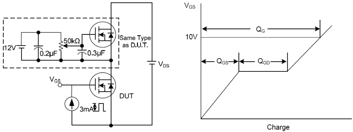
图12. 栅电荷测试
