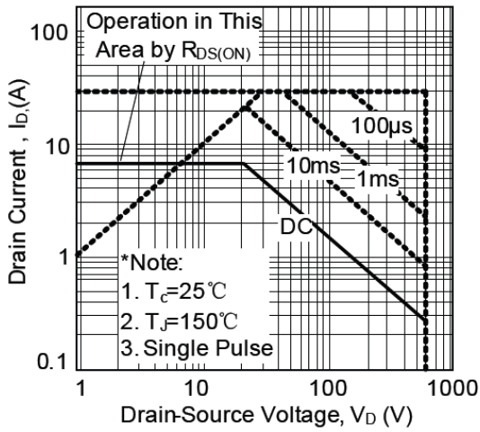
图7. 最大安全工作区 Fig. 7 Maximum Safe Operating Area
