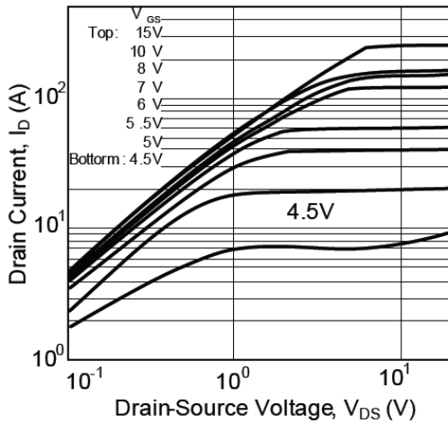
图1. 输出特性曲线 Fig. 1 On-State Characteristics
