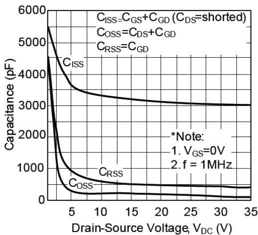
图5. 电容特性曲线 Fig. 5 Capacitance Characteristics
