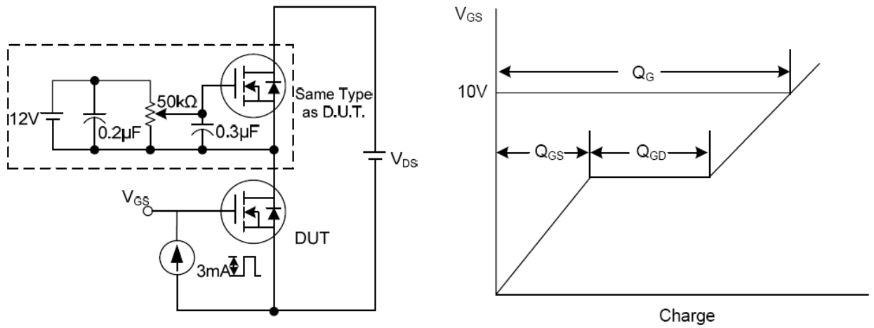
图12. 栅电荷测试
