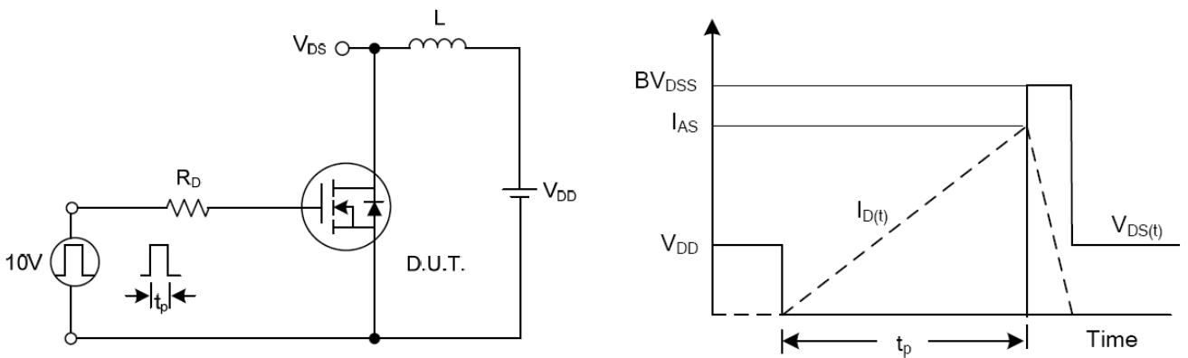
图13. 雪崩能量测试
