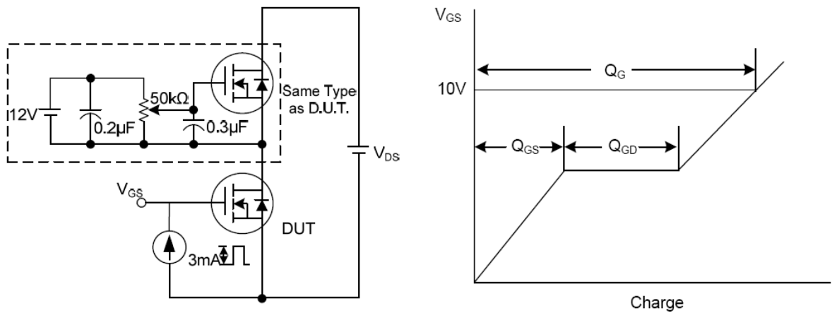
图12. 栅电荷测试
