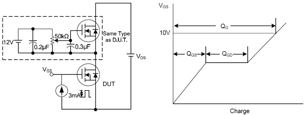
图12. 栅电荷测试
