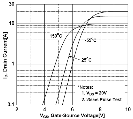
图2. 传输特性曲线
