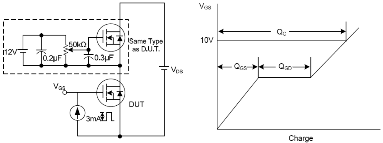
图12. 栅电荷测试
