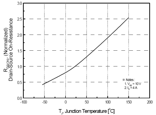
图4. 导通电阻随温度变化曲线
