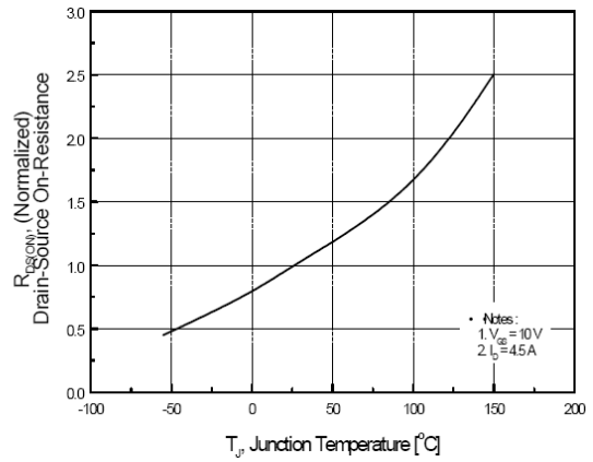
图4. 导通电阻随温度变化曲线
