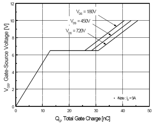
图6. 栅电荷特性曲线
