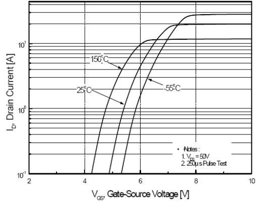
图2. 传输特性曲线
