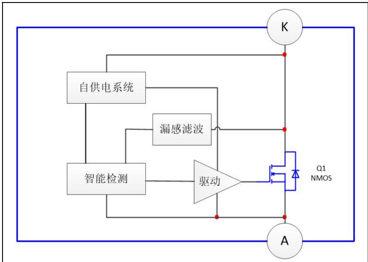
电路结构方框图
