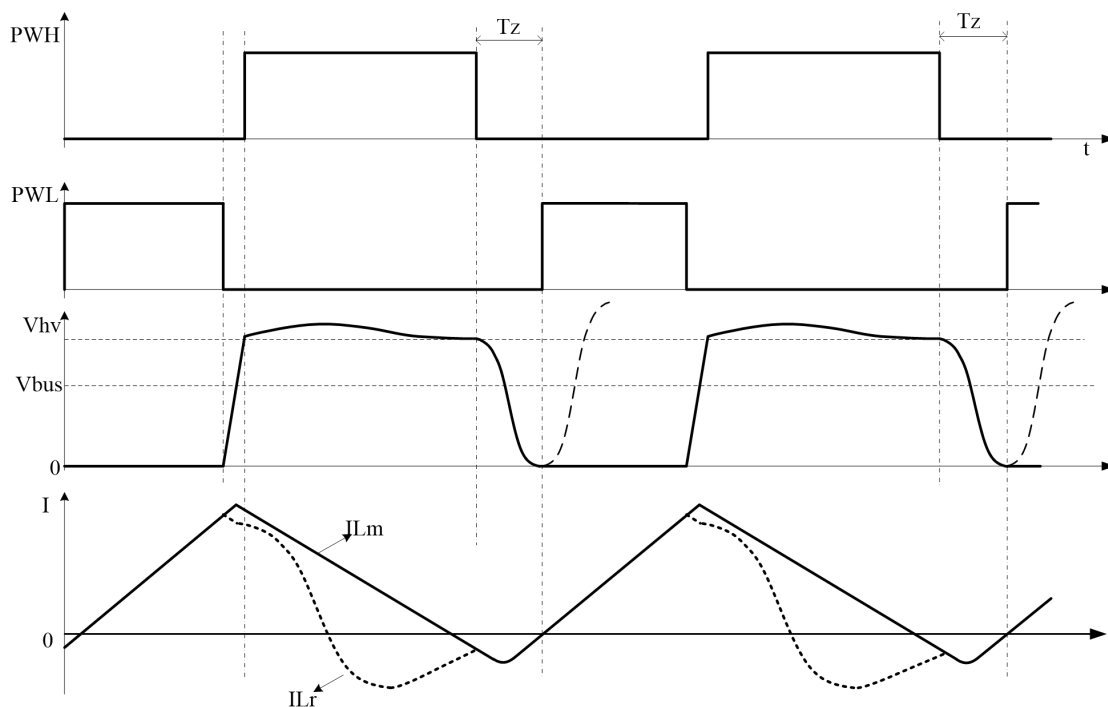
工作波形图
