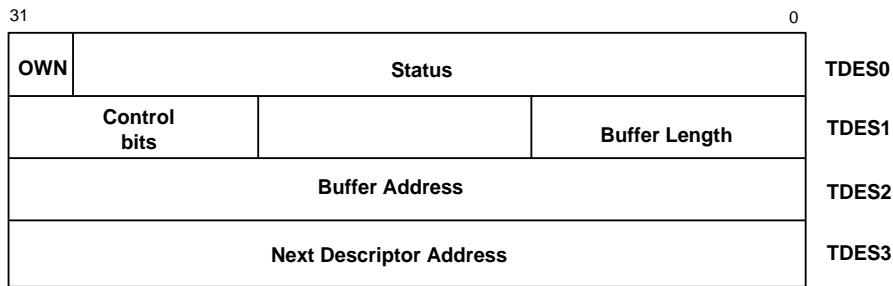
Transmit Descriptor Format
