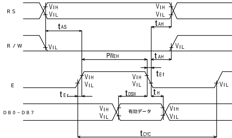
図1 ライト動作
