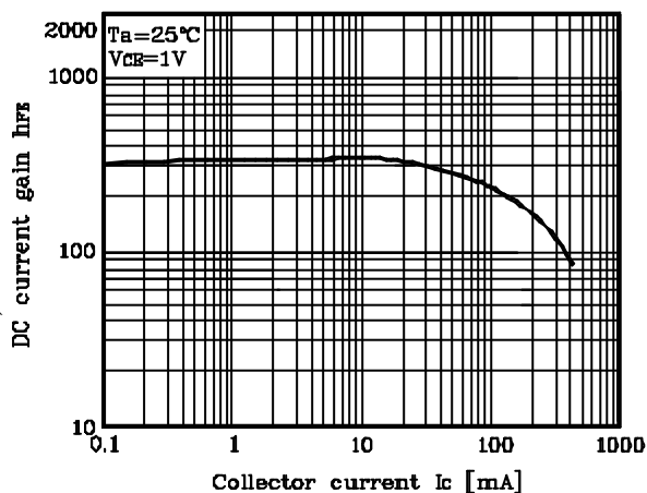
Fig. 3 h_{FE} - I_C
