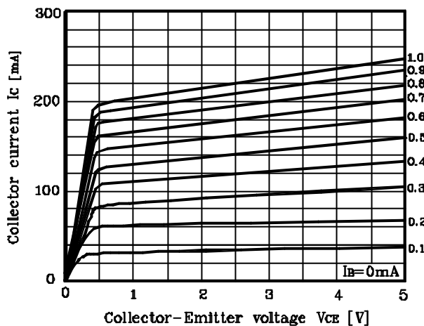
Fig. 4 I_C - V_{CE}
