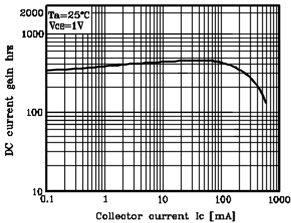
Fig. 3 h_{FE} - I_C
