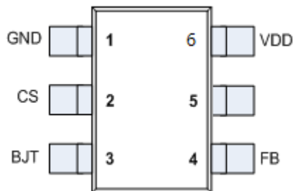
SOT23-6
