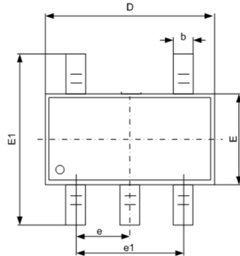
SOT23-5
