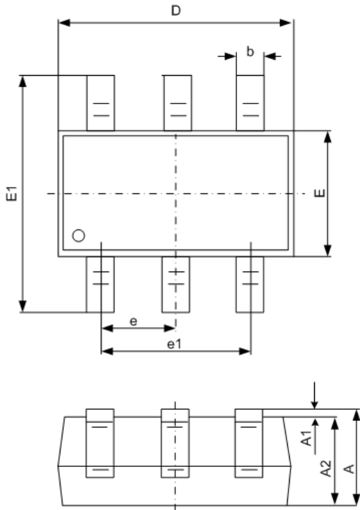
SOT23-6
