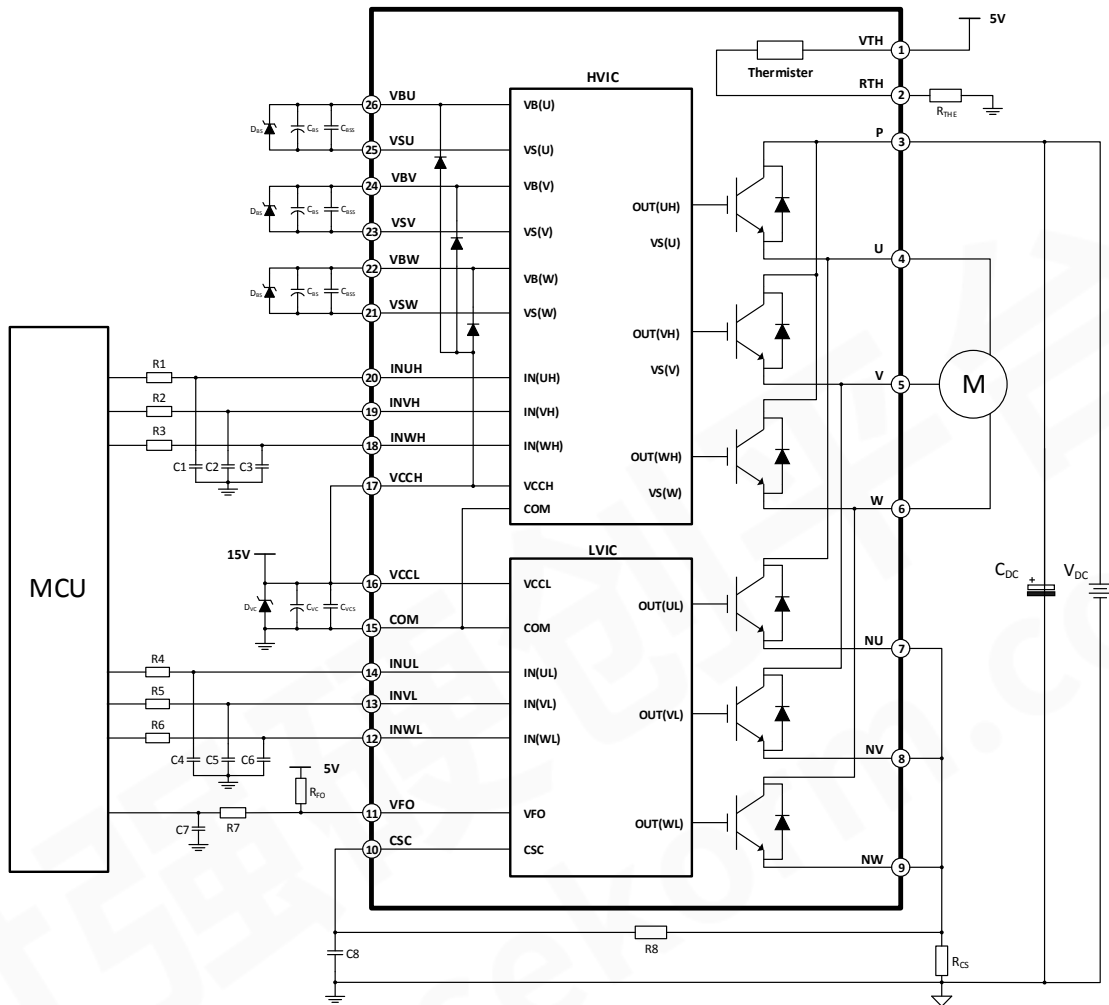
图 10 DPM15C60BG2 典型应用线路
