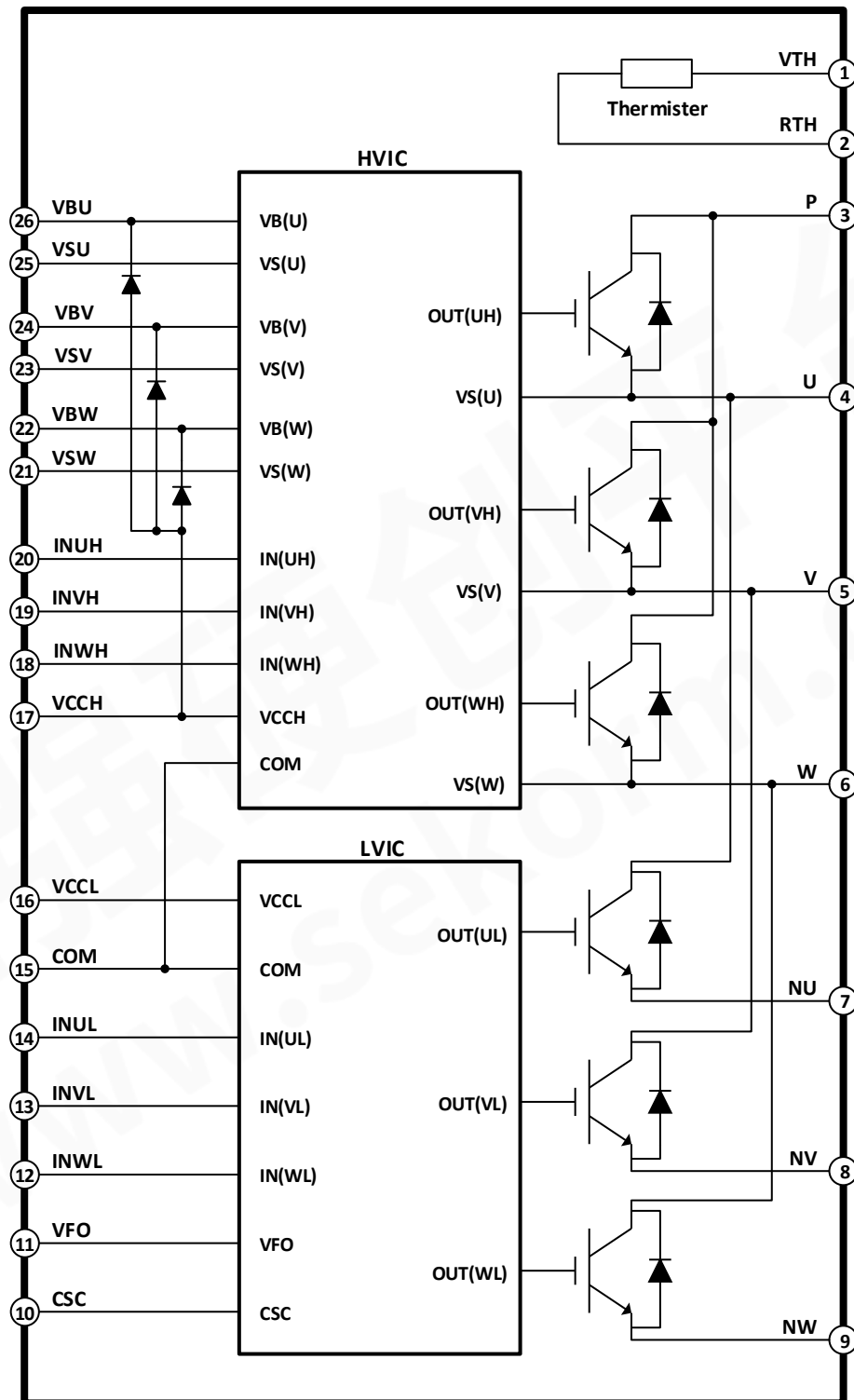
图 1 DPM15C60BG2 功能框图
