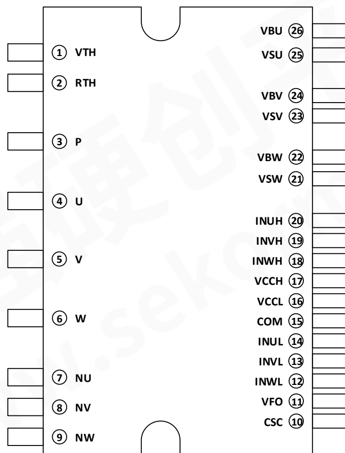
图 2 引脚排列图
