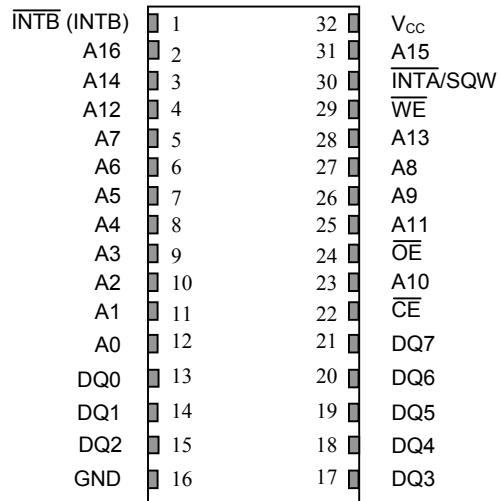
DS1486 128k x 8
