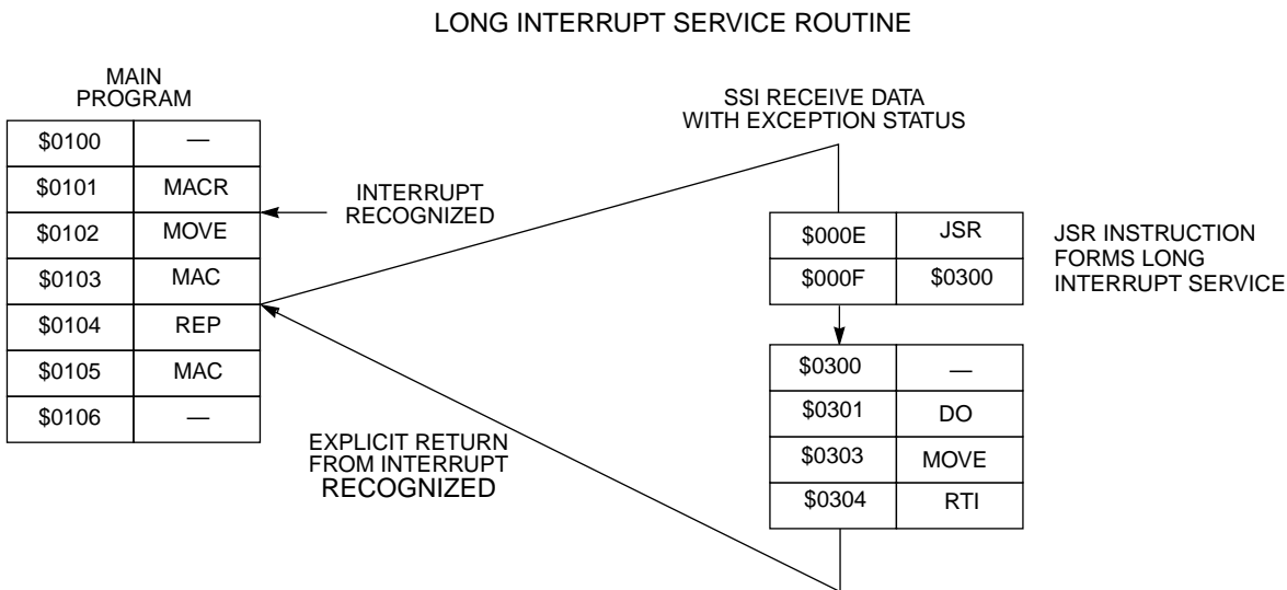
(b) DSP56K Long Interrupt
