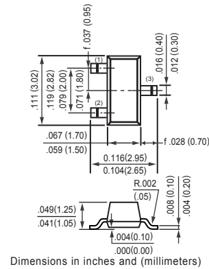
SOT-23-3L
