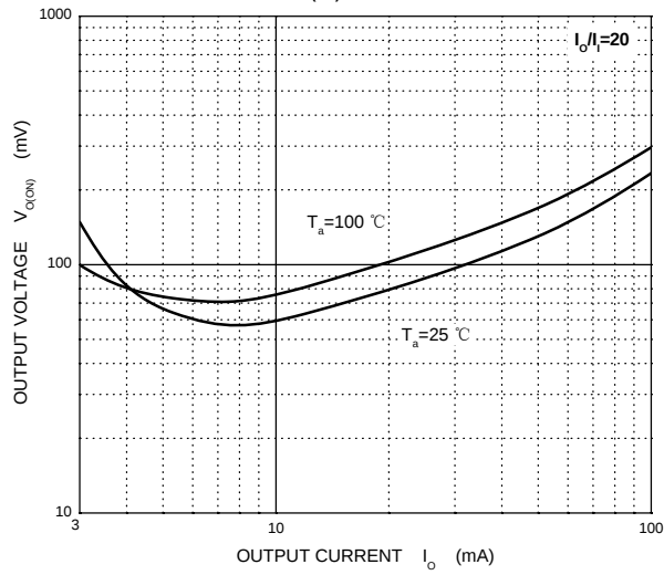
V_{OL(on)} — I_O
