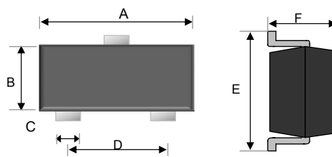
SOT-323
