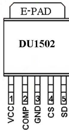
TO252-5 封装
