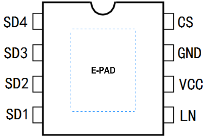
ESOP8 封装
