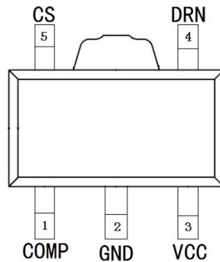
SOT89-5 封装
